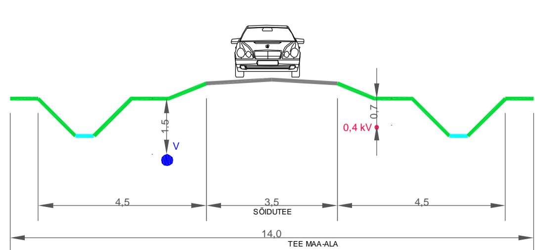
TEE RISTPROFIIL M 1:100
