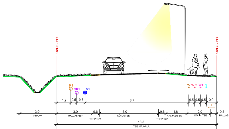
TEE TÕUPRISTPROFIIL 13,5 m. KRAAV PAIKNEB KINNISTUL.
