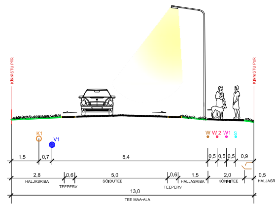
TEE TÕUPRISTPROFIIL 13,5 m. KRAAV PAIKNEB KINNISTUL.
