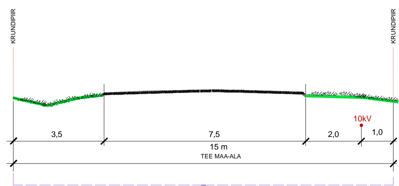
T-21111 Tehumardi-Kogula TEE RISTPROFIIL
