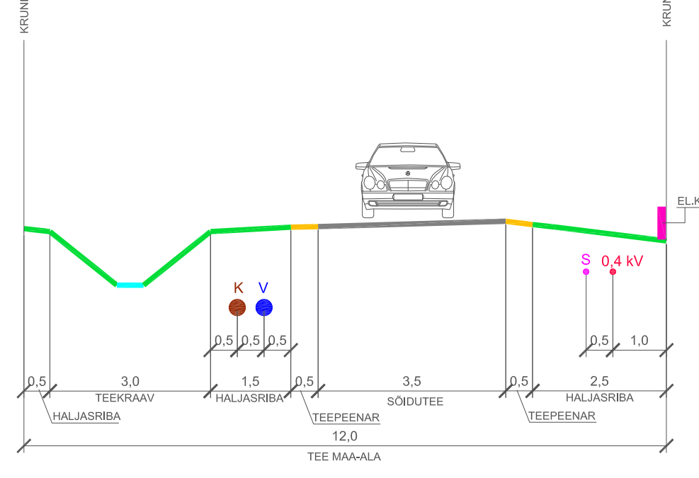
KRUNDIDE JUURDEPÄASUTEE RISTPROFIIL A-A M 1:100
