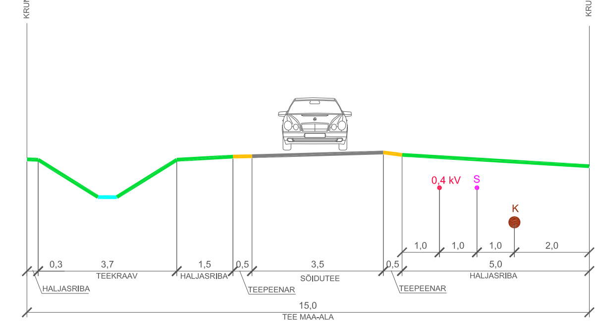
LAISELJA TEE SOOVITUSLIK RISTPROFIIL B-B M 1:100
