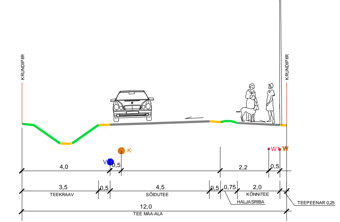
MUSTIKA JA MAASIKA MÜ. DETAILPLANEERINGU TEEDE TÕÜPRISTPROFIIL
