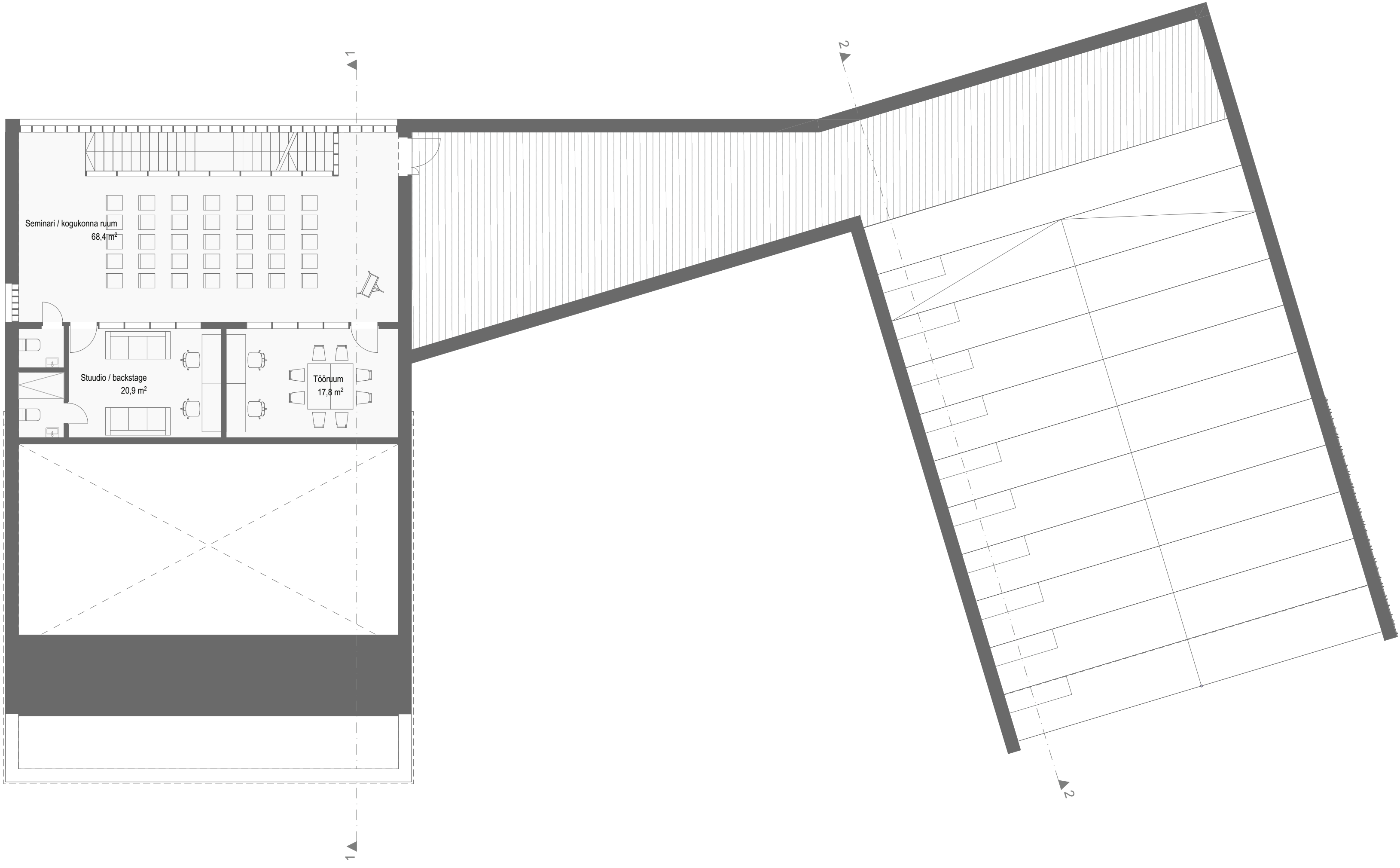
2. korrus M1:100
