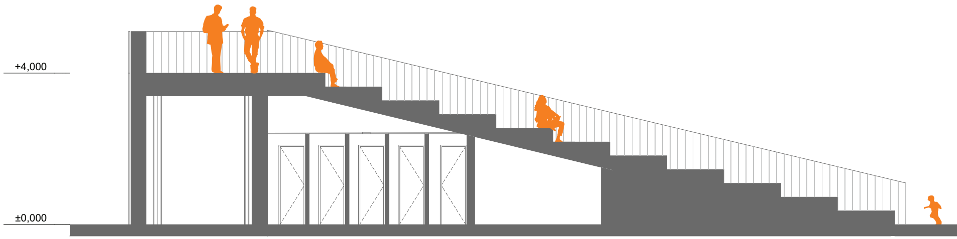
Lõige 2-2 M1:100
