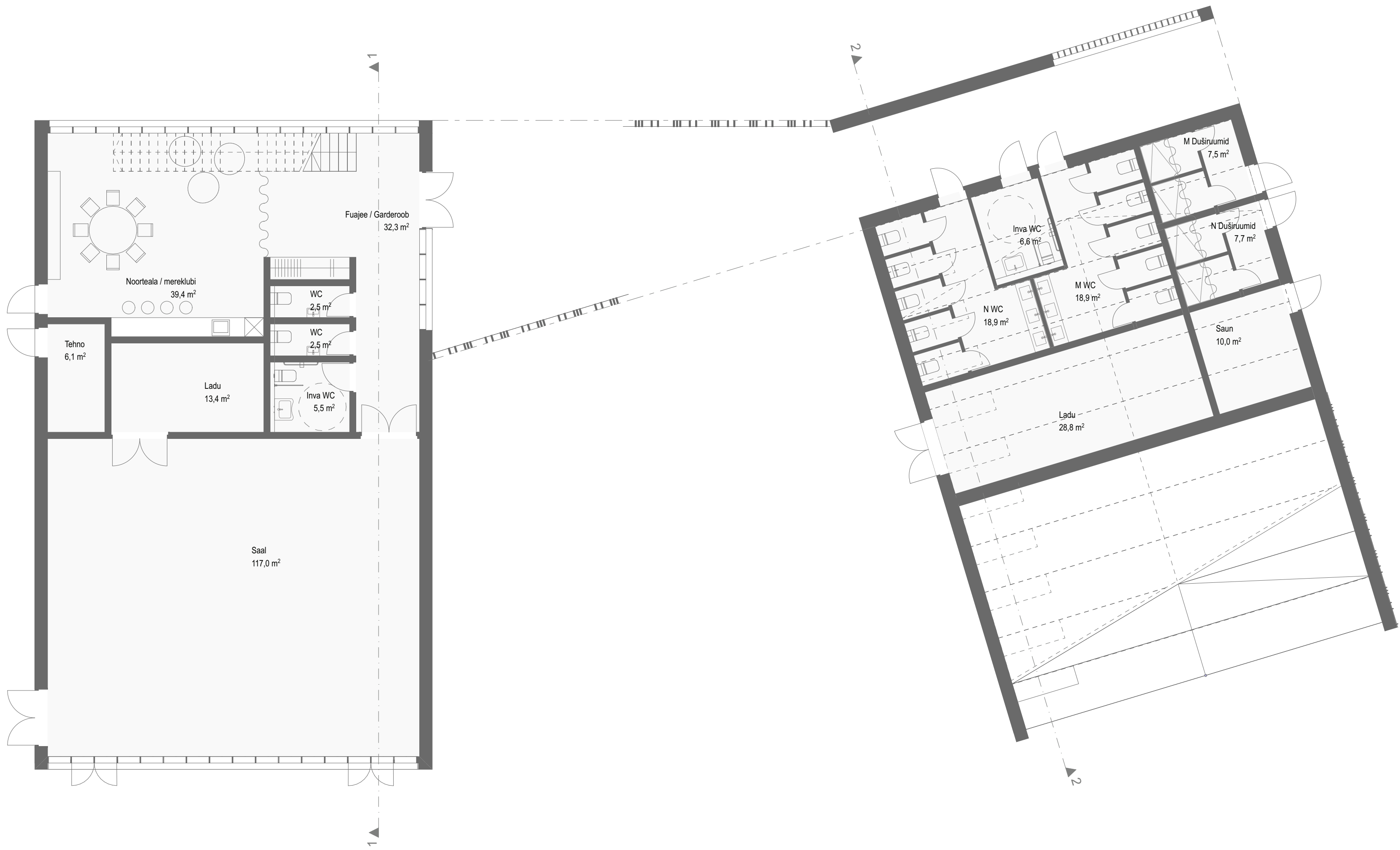
1. korrus M1:100
