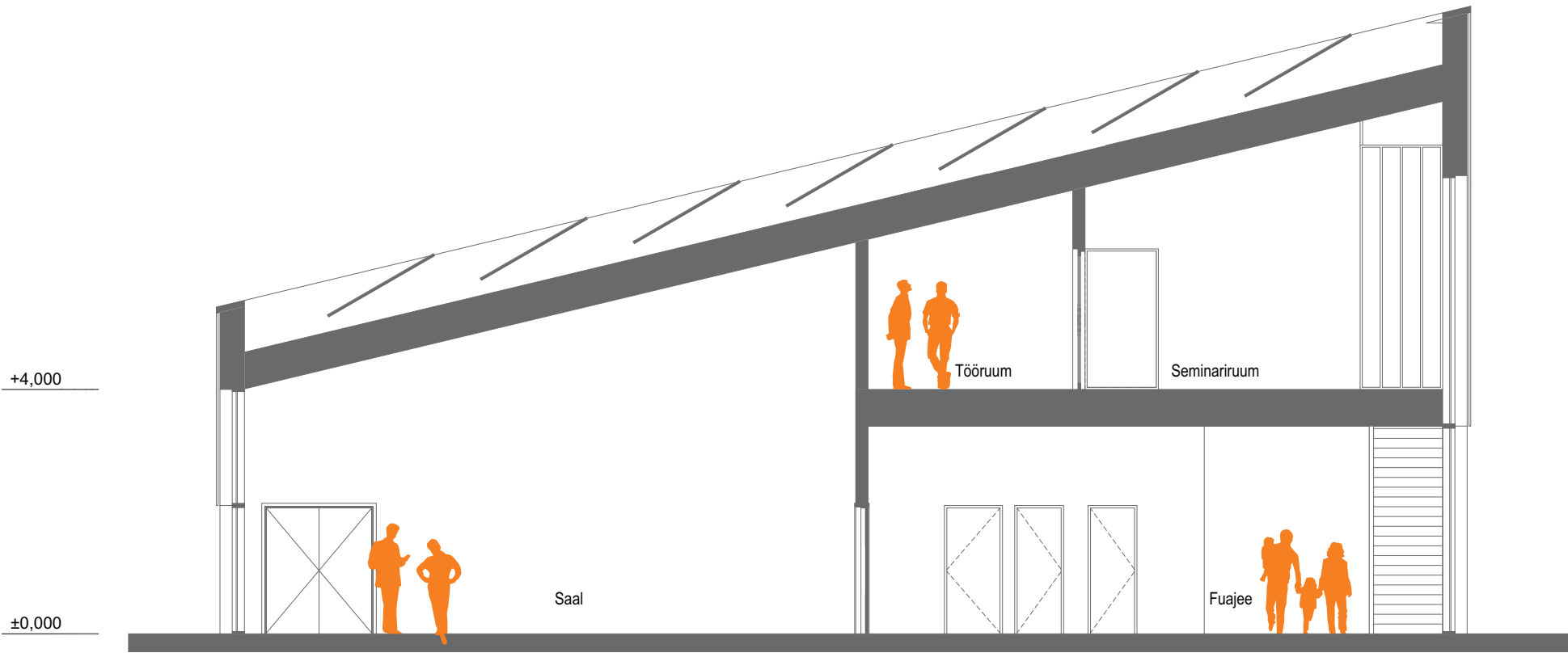
Lõige 1-1 M1:100
